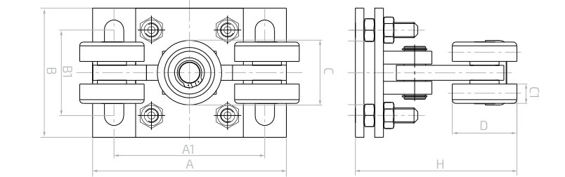
Wózek jezdny 80 rolki z tworzywa Cantilever gate carriage / Роликовая каретка / Laufrollenbock
