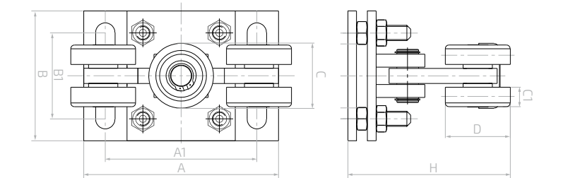
Wózek jezdny 70 rolki stalowe Cantilever gate carriage / Роликовая каретка / Laufrollenbock
