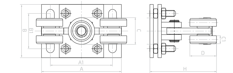
Wózek jezdny 70 rolki z tworzywa Cantilever gate carriage / Роликовая каретка / Laufrollenbock
