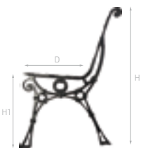
Noga aluminiowa do ławki Bench leg / Аллюминиевая нога скамьи / Bankfuß
