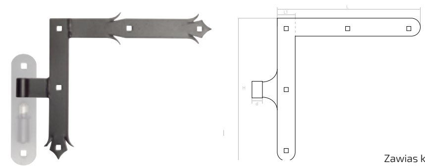
Zawias kątowy ozdobny Hinge / Петля / Scharnier
