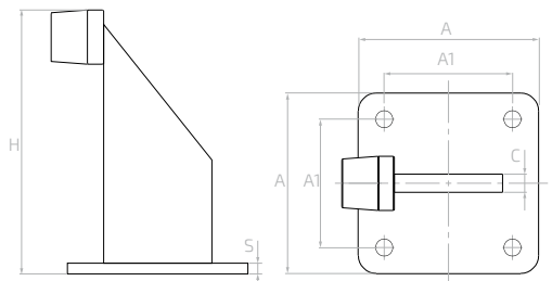
Zderzak zewnętrzny z płytką Gate stopper / Наружный отбойник с креплением / Torstopper mit Platte
