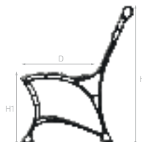
Noga aluminiowa do ławki Bench leg / Аллюминиевая нога скамьи / Bankfuß
